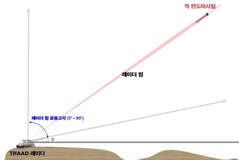
[ THAAD 레이더 빔 운용고각 ]
