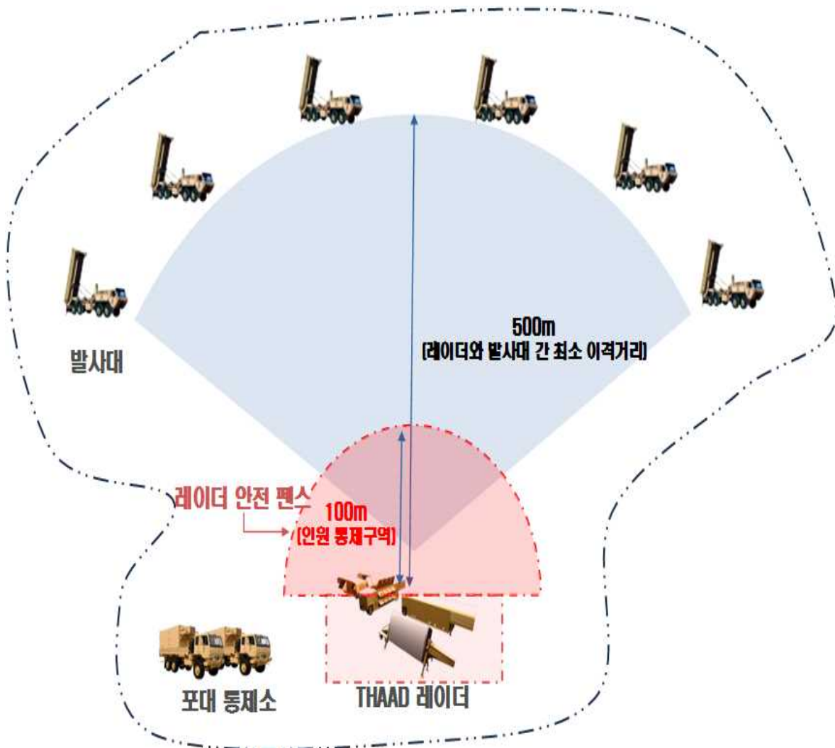
[ THAAD 포대의 장비 배치 개념도 ]
